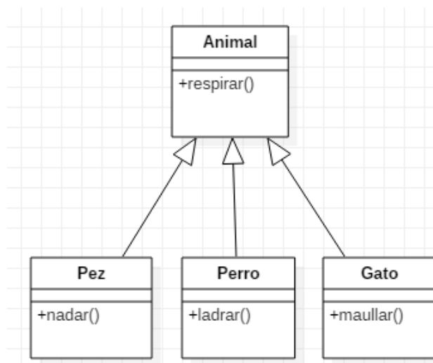
Ejemplo de herencia
