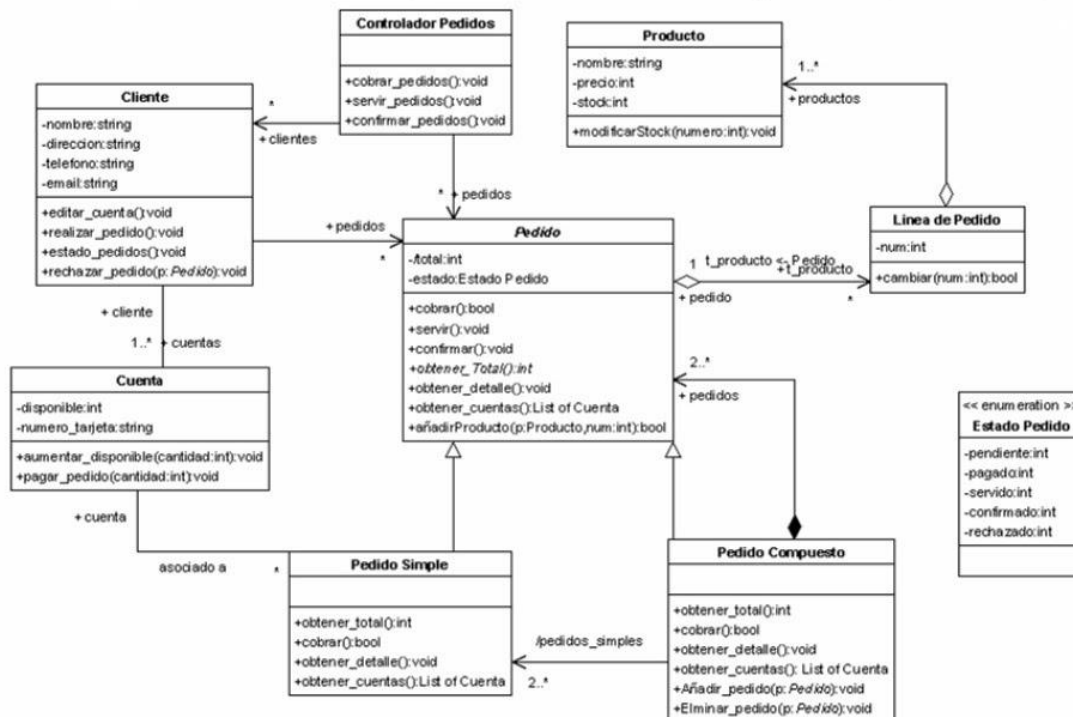
Ejemplo 3. Diagrama de clases de pedidos de productos en línea.
