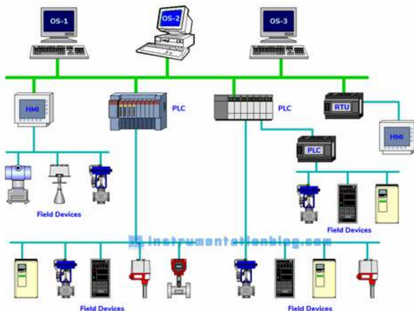
Figura 6: Esquema de un DCS. Fuente: InstrumentationBlog (2025).
